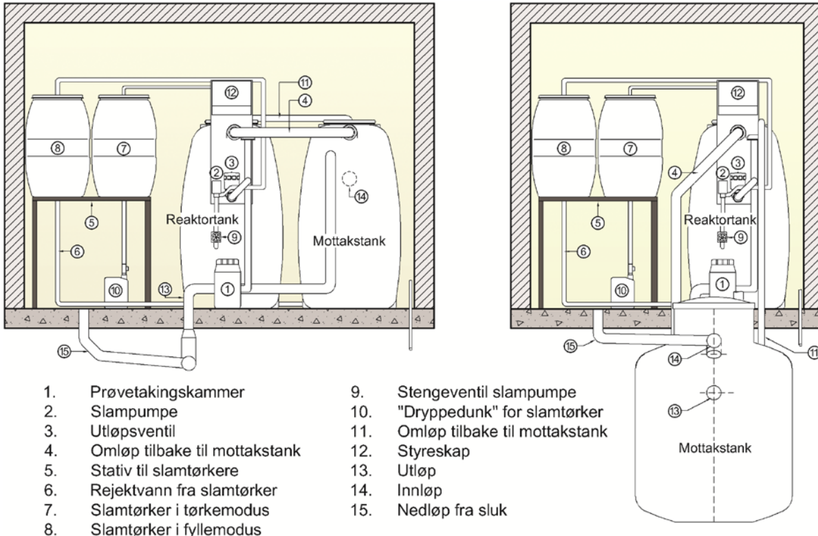
Figur 1. Skisse av henholdsvis Biovac FD 5 MG med mottakstank plassert innendørs, og Biovac FD 5 med nedgravd mottakstank.
